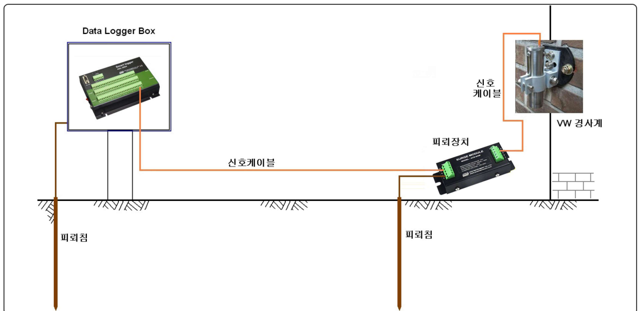
[모델 ACE-SAM 피뢰장치의 구성도]
