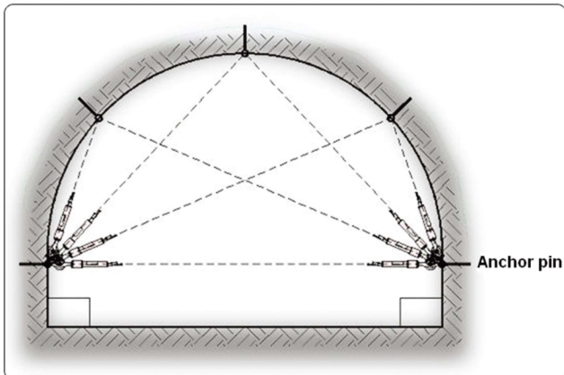
[터널 내공 변위계 측정 개념도]
